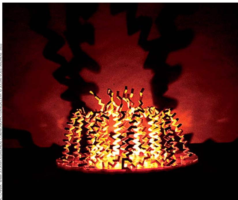
В СВЕТОСОБИРАЮЩИХ КОМПЛЕКСАХ — «АНТЕННАХ» ФОТОСИНТЕЗА — СОСРЕДОТОЧЕНО ДО 90% ХЛОРОФИЛЛА
